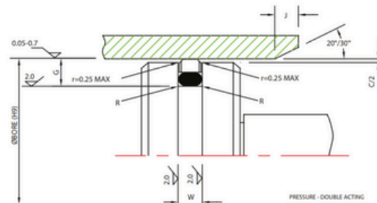
F100B Piston Seal
